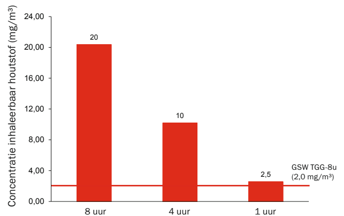
Toetsing blootstelling inhaleerbaar houtstof aan grenswaarde
