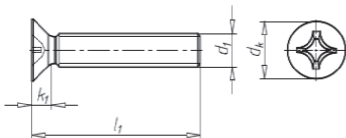
NX 100331 - L1 = 70 mm d1 = M6
