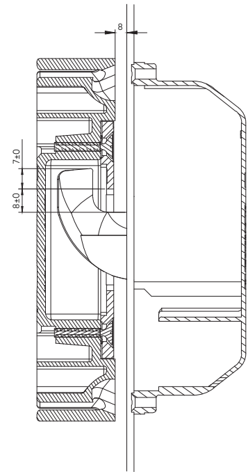
Detail sluithaak in sluitkom
