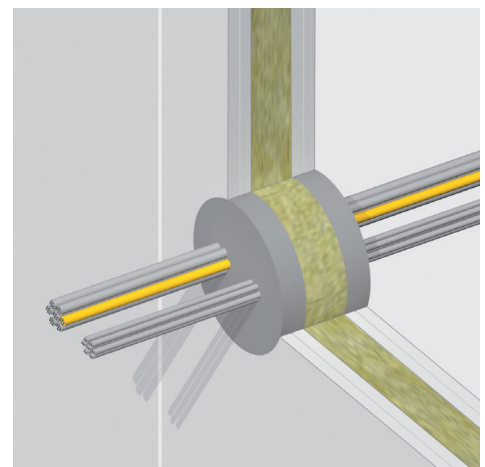
Losse kabels en E-leidingen door muur
