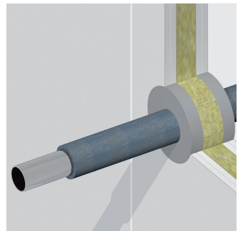
Metalen buis voorzien van Armaflex isolatie
