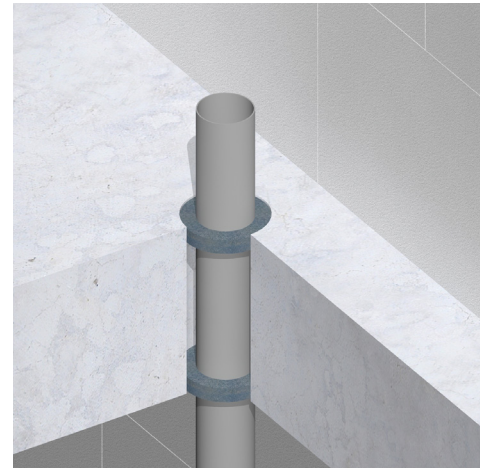
Kunststof buis tot maximaal Ø 125 mm
